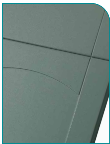
Altea Seff Pistacho Radio: R4 Grosor: 19/22 mm. Profundidad: 1.5 mm. Marco: 6 cm.
